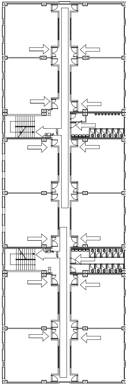
PLANTA PRIMERA ESCALA: 1/200
